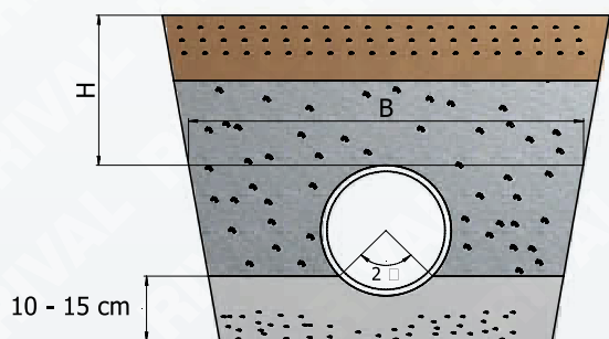
Dimensiones de la zanja
