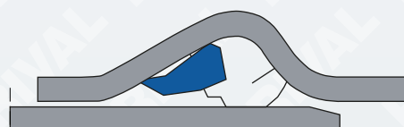
Compresión del labio de sellado
