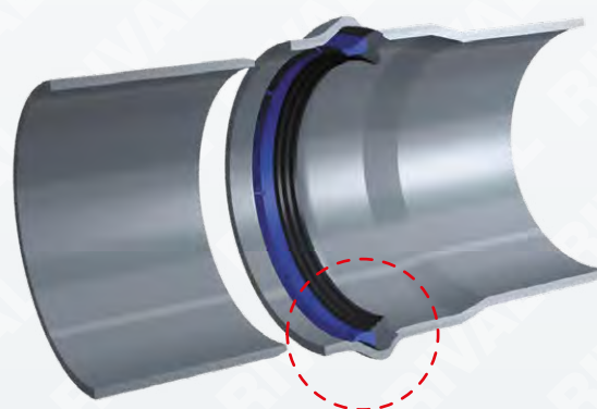
Junta Tipo FORSHEDA 576 Anger-Lock
