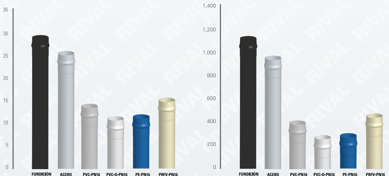
Golpe de ariete (P) en bares
