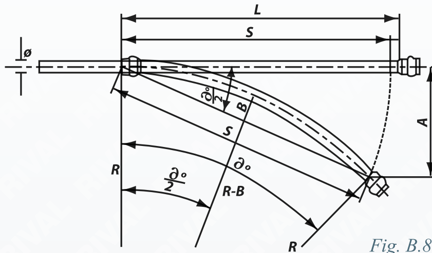
Fig. B.8 - Dimensiones relativas a la curvatura del tubo
