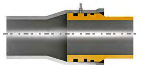
Espiga y enchufe con doble aro de goma
