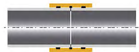
Unión tipo REKA con doble anillo de goma.
